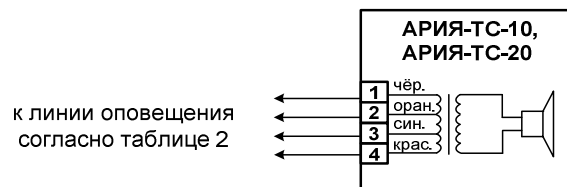
Рис.1. Схема подключения.
