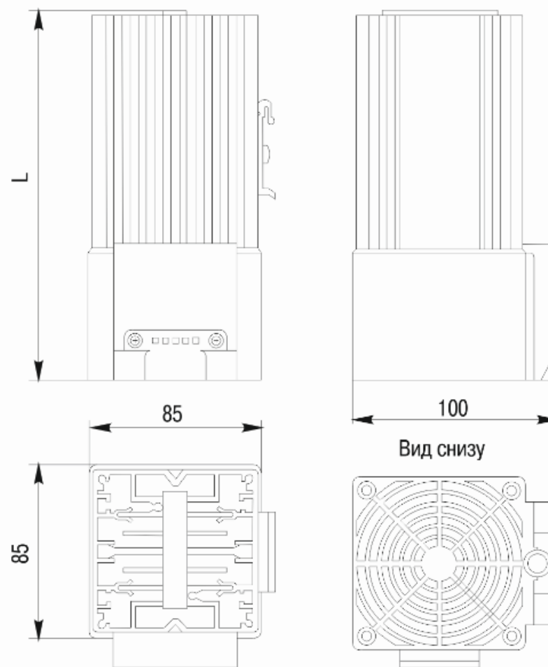
Рисунок 1 Габаритные размеры обогревателей
