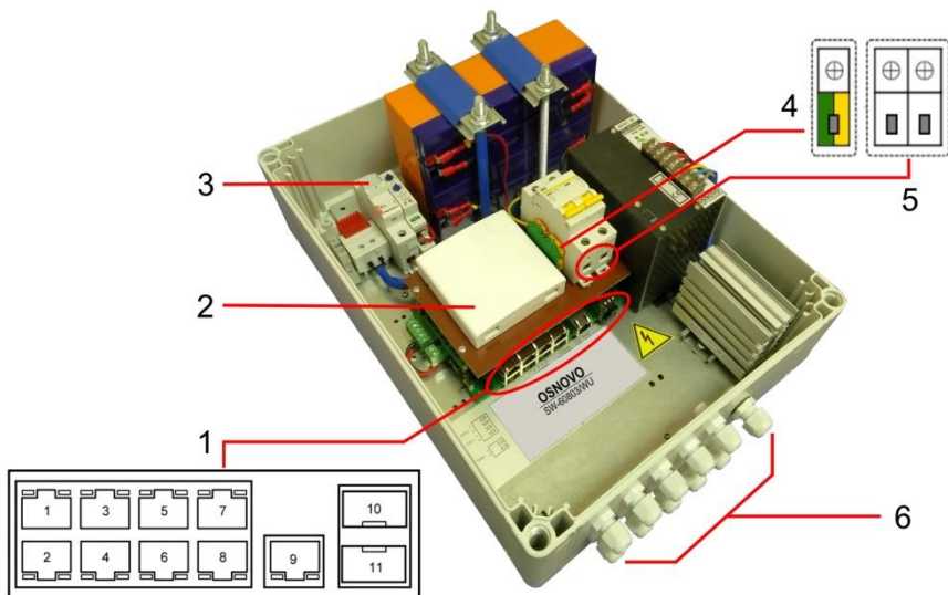
Рис. 4 Подключение коммутатора SW-60812/WU
