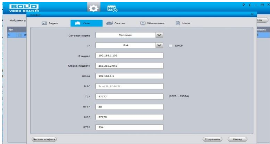
Рисунок 12.2 – Изменение IP-адреса видеокамеры с помощью утилиты «BOLID VideoScan»
