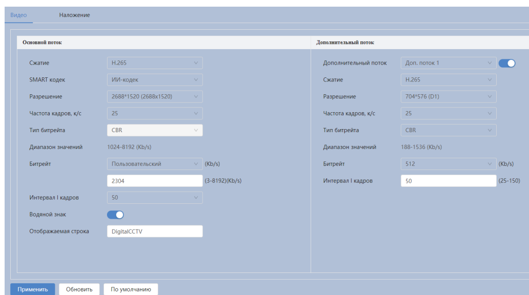
Рисунок 7.39 – Вкладка «Видео»
