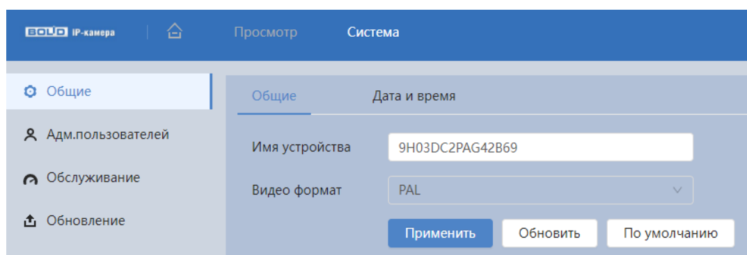
Рисунок 7.70 – Вкладка «Общие»
