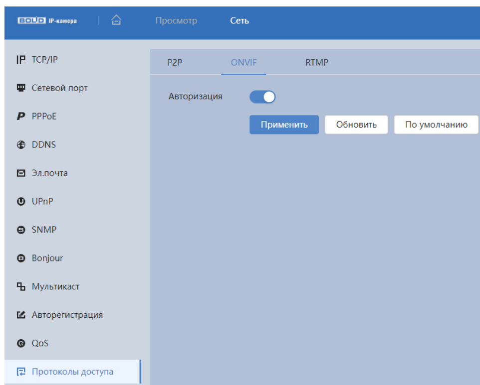
Рисунок 8.20 – Вкладка «ONVIF»
