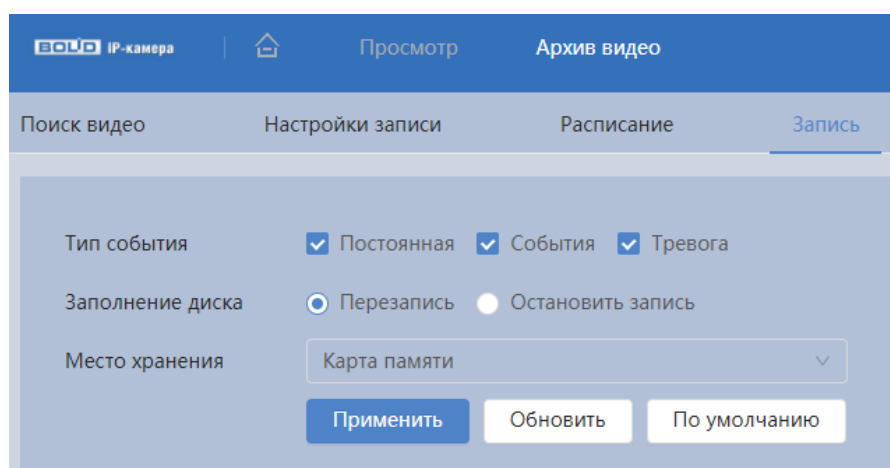
Рисунок 7.95 – Вкладка «Запись»
