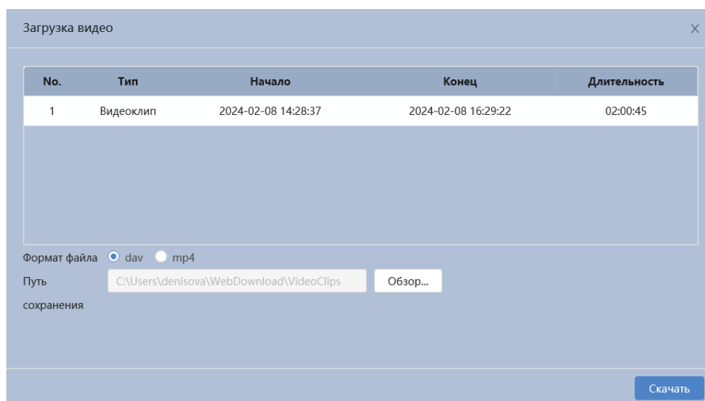
Рисунок 7.91 – Загрузка видео
