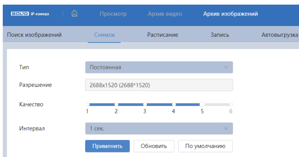
Рисунок 7.98 – Вкладка «Снимок»
