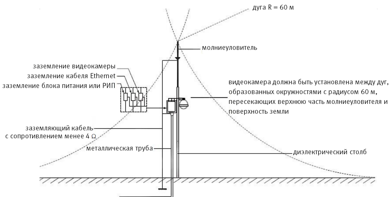
Рисунок 6.13 – Установка молниеотвода
