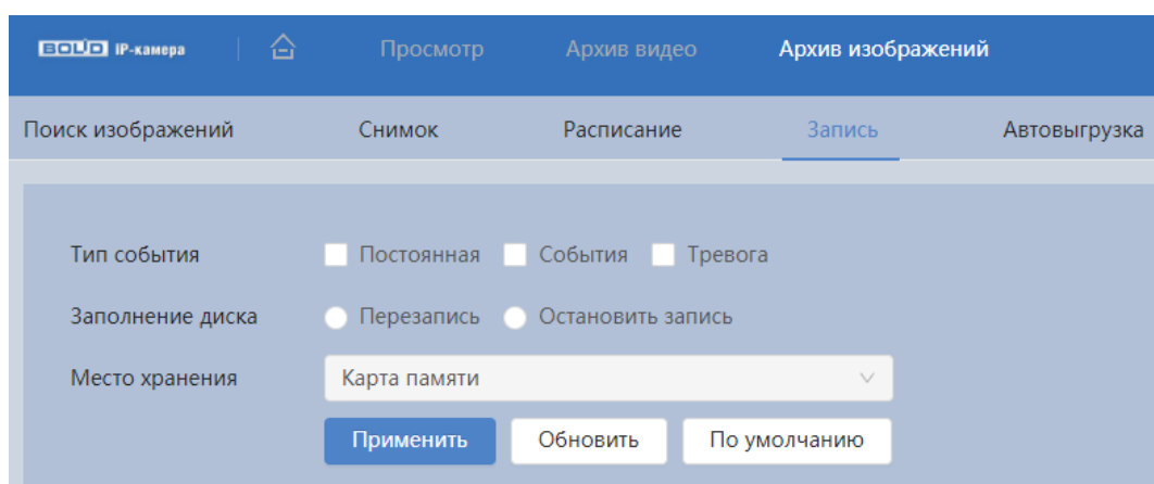
Рисунок 7.101 – Вкладка «Запись»
