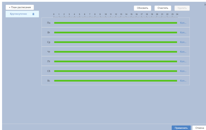
Рисунок 7.59 – Вкладка «Расписание»
