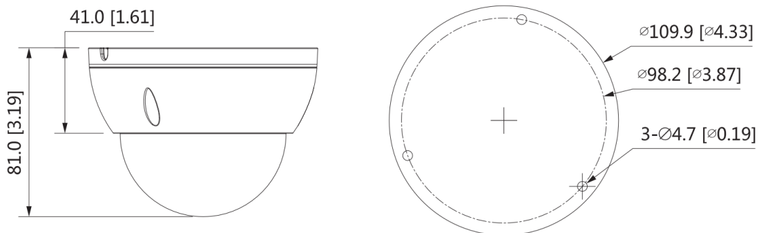
Рисунок 5.1 – Габаритные размеры видеокамеры
