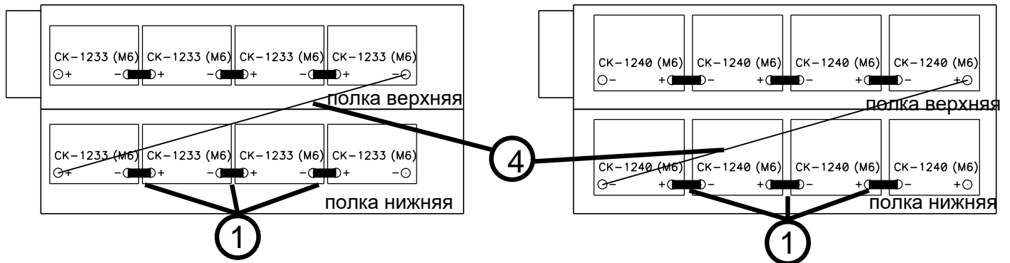
Стеллаж MBS-01 для 40 Ач Типовое расположение АБ.
