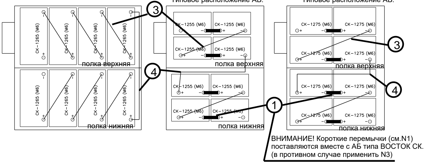
Стеллаж MBS-03 для 65 Ач Типовое расположение АБ.
