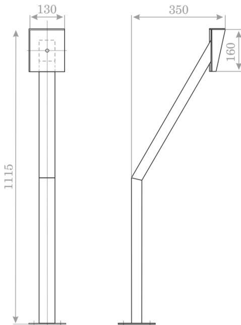
Рисунок 2. Общий вид стойки
