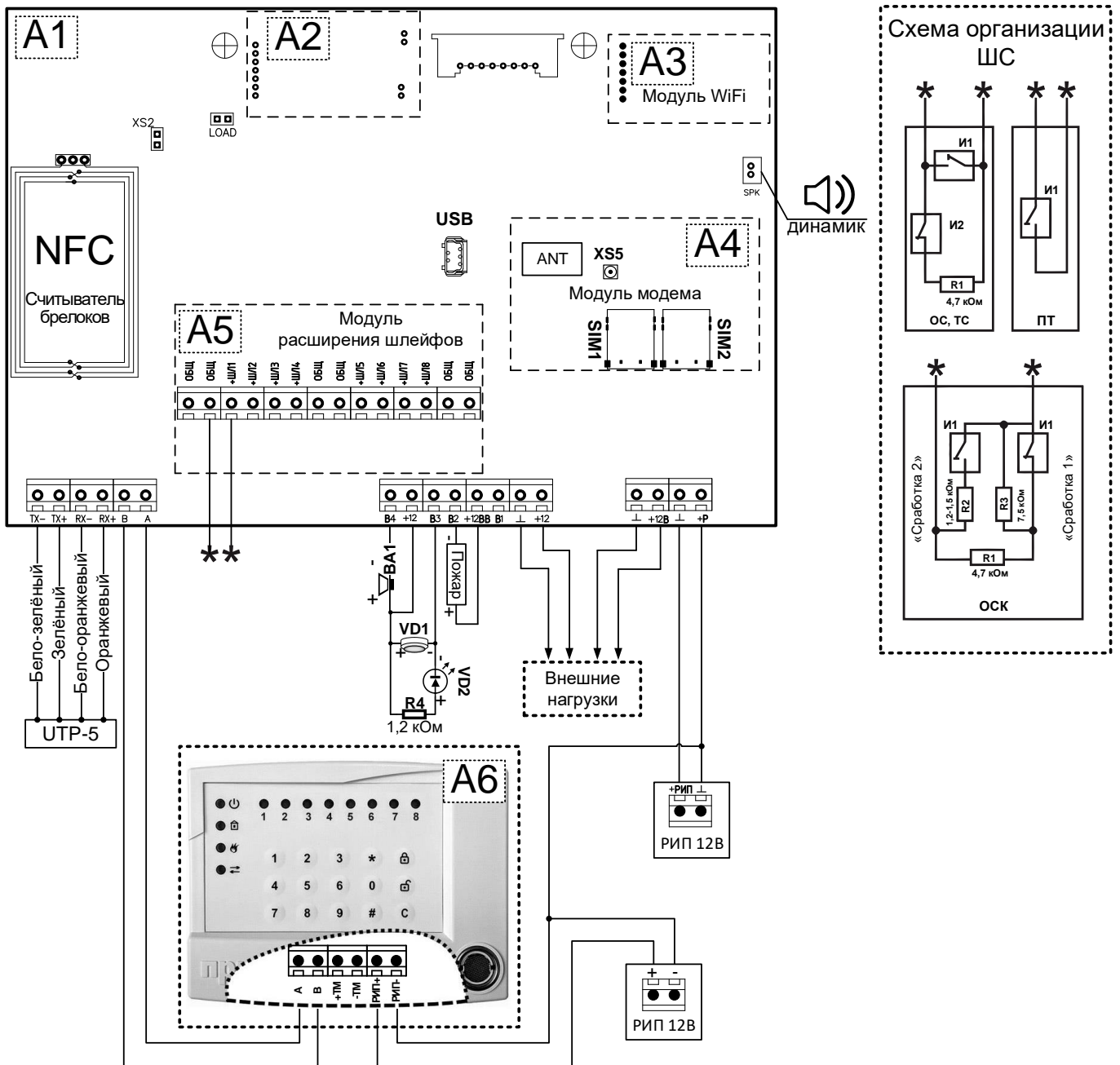
Рисунок 6 – Схема подключения прибора Приток-А-КОП-01(8)
