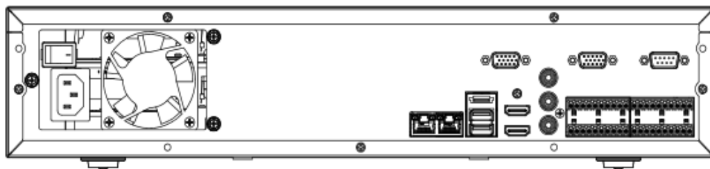
Рисунок 4.2.1 Схема обозначения портов.
