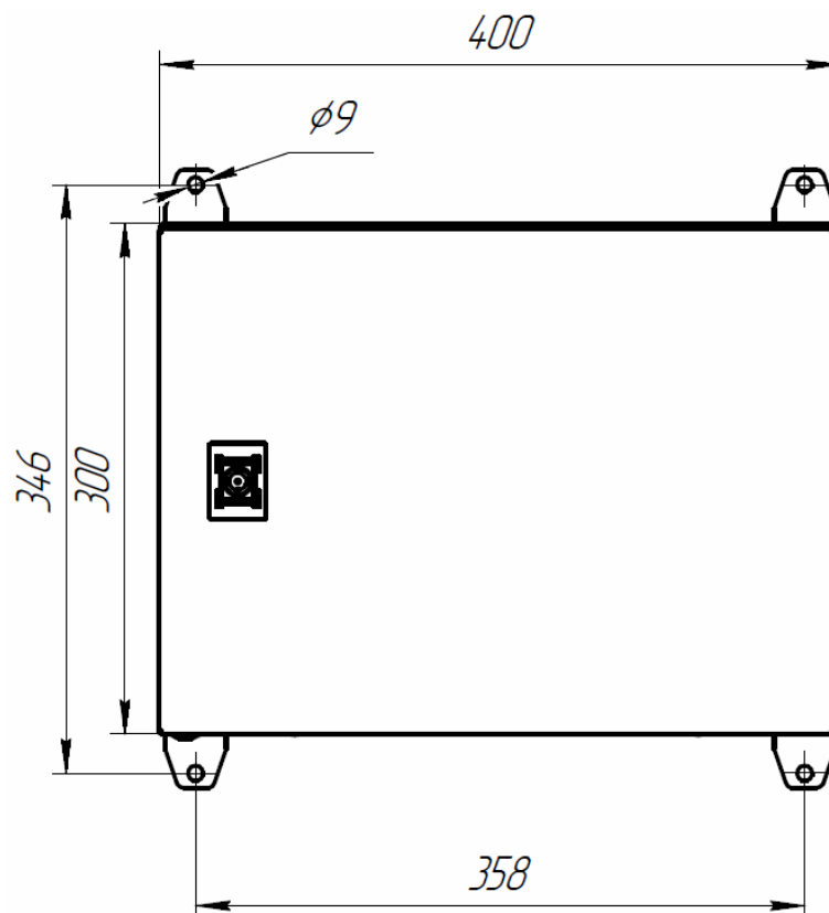
Рисунок 14. Расположение крепежных элементов коммутатора
