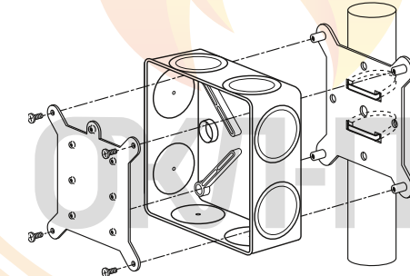
Рис. 12. Монтаж к трубным конструкциям
