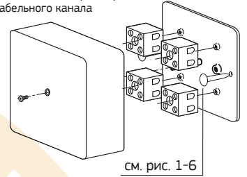
Рис. 13. Монтаж и сборка коробки для кабельного канала
