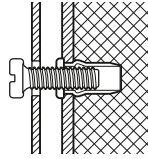
Рис. 4. Сэндвич-панели
