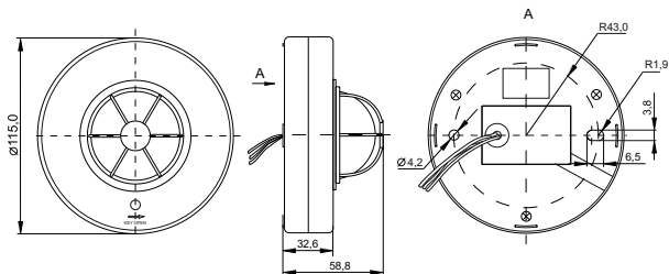
Рисунок 3 – Габаритные размеры
