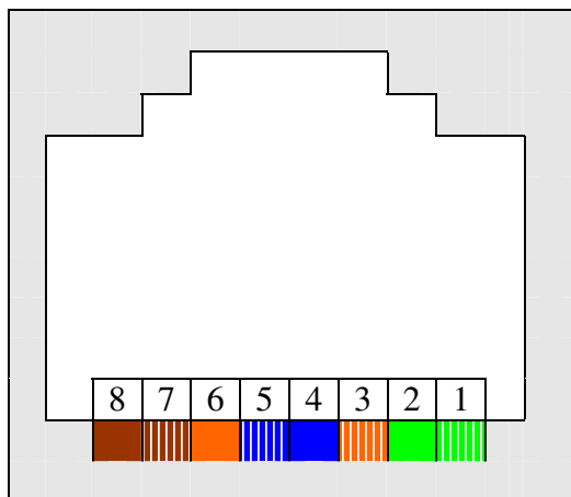
Рис. 3. Нумерация контактов
