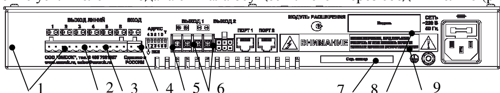
Рис. 2. Нижняя панель модуля расширения. 1 – выход линий (коммутируемый), 2 – резервный вход коммутатора, 3 – переключатель адреса, 4, 5 – некоммутируемые выходы модуля расширения, 6 – порт связи, 7 – клемма защитного заземления, 8 – сетевой предохранитель, 9 – соединитель сетевого питания.
