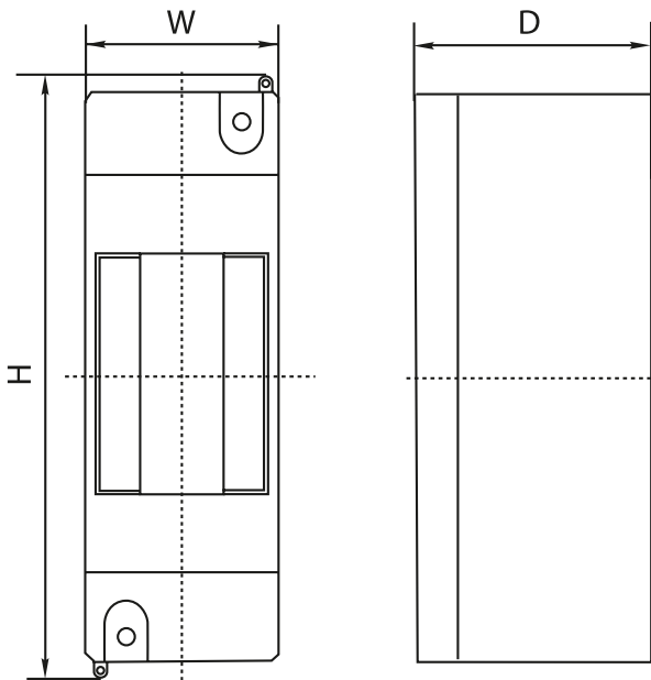
Рис. 1 - Габаритные размеры корпусов КМПн
