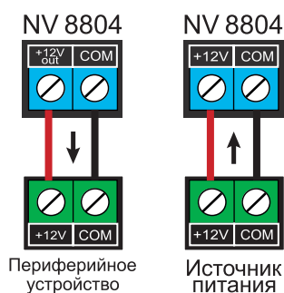
Рисунок 1. Подключение питания
