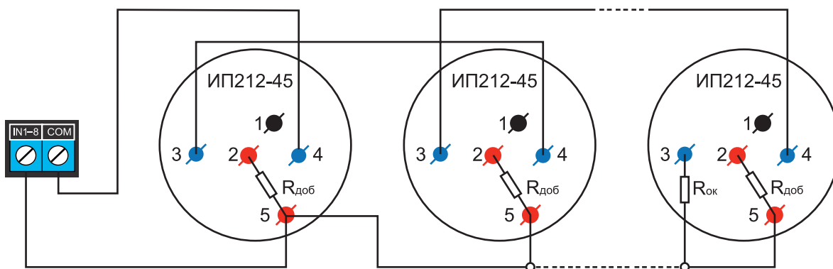
Рисунок 2. Схема подключения ИП212-45 к пожарному входу NV 8804 с добавочными и с оконечными резисторами
