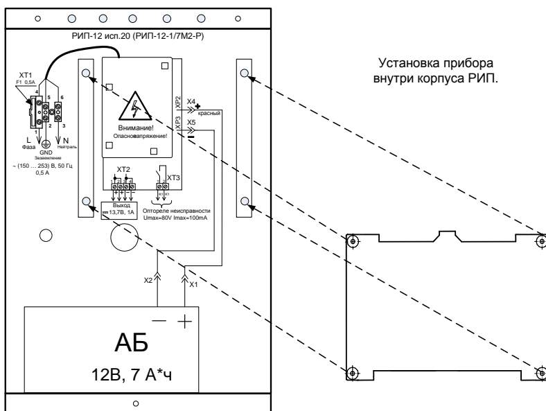
Рисунок 3. Установка прибора внутри корпуса РИП.
