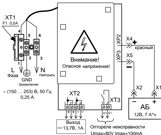
Рисунок 2. Схема подключения РИП-12 исп.20 (РИП-12-1/7М2-Р)
