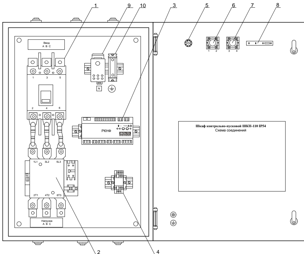
Рисунок 2. Внутреннее устройство шкафа
