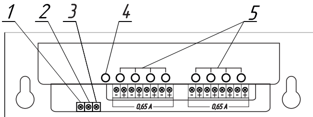
Схема подключения ББП FE-1250 V.8 MAX
