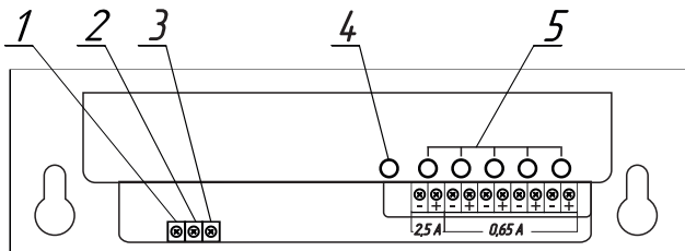
Схема подключения ББП FE-1250 V.5 MAX
