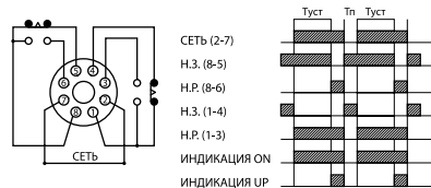
Рисунок 14. Схема работы реле времени PB2, PB3
