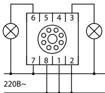
Рисунок 11. Электрическая схема подключения реле PB1, PB2, PB3, PB4
