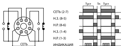
Рисунок 13. Схема работы реле PB1 (в режиме работы В)
