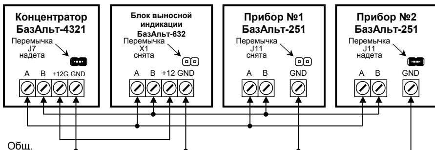
Рисунок 1 – Пример подключения приборов к концентратору
