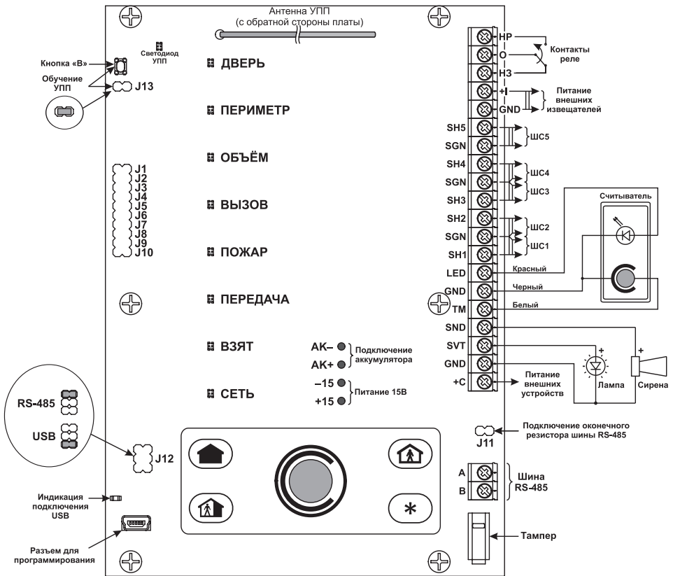
Рисунок 8 – Монтажная схема прибора
