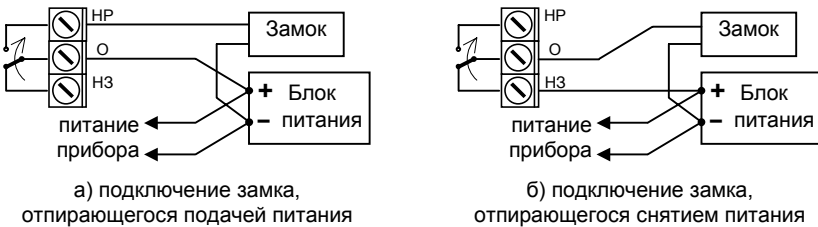
Рисунок 7 – Подключение электрического замка
