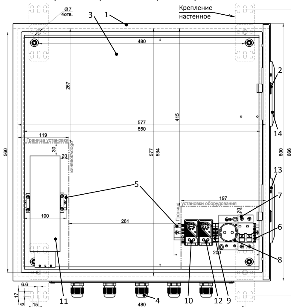
Рисунок 1 – Устройство шкафа
