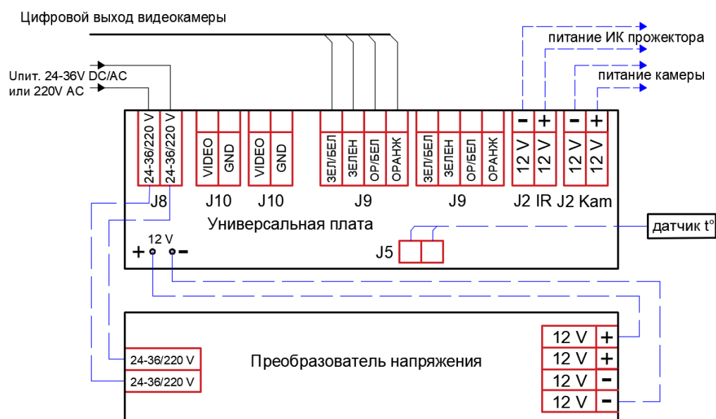
Рисунок 2 – Схема внешних подключения видеокмеры. Синей пунктирной линией указаны внутренние цепи.
