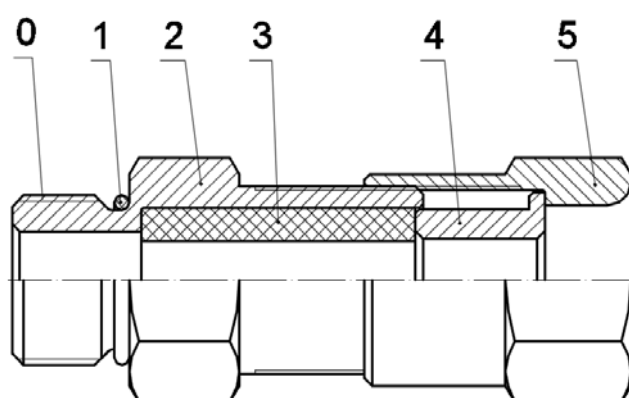
KBH – для монтажа открытого кабеля
