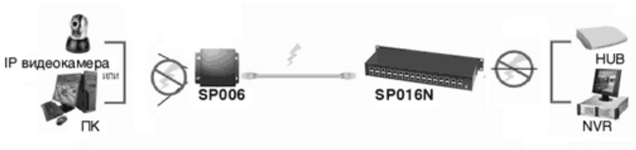
Рис.2 Подключение SP016N .
