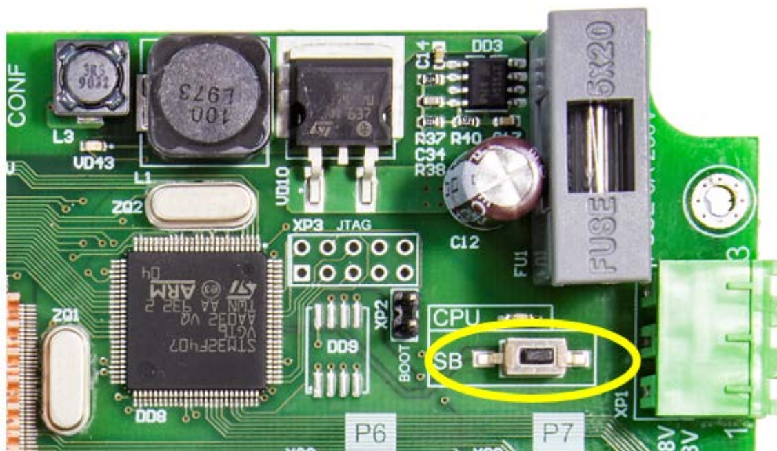
Рисунок 11. Кнопка сброса настроек коммутатора на заводские установки
