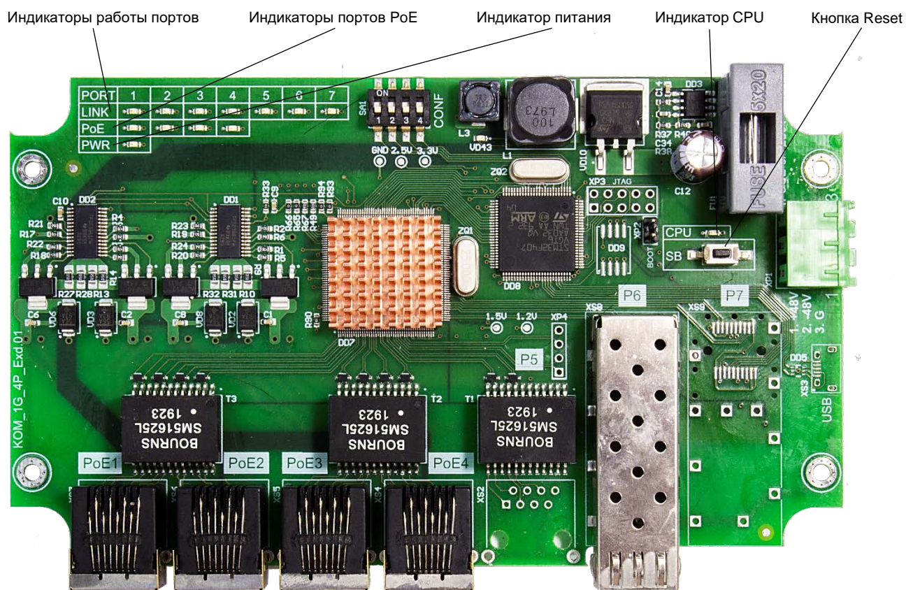
Рис. 4. Расположение элементов Релион-SW-1G-4PoE+/140W
