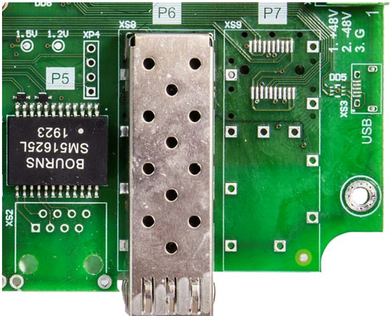
Рисунок 6. Фото порта SFP коммутатора
