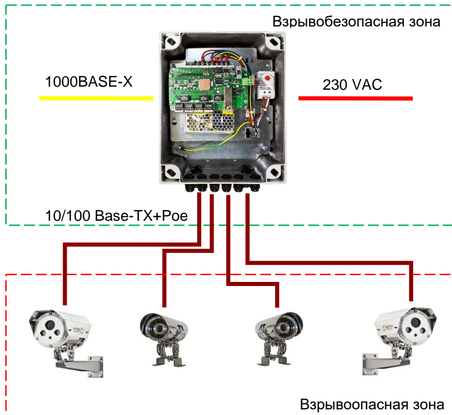
Рисунок 1. Типовые схемы подключения Релион-SW-1G-4Poe+/140W по оптическому кабелю
