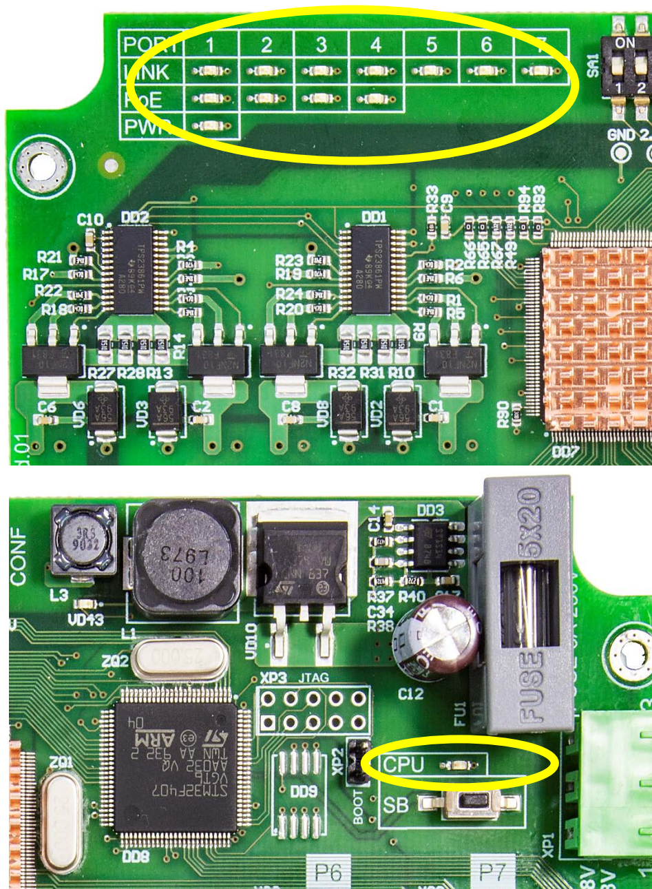
Рисунок 10. Расположение элементов индикации и настройки на плате коммутатора
