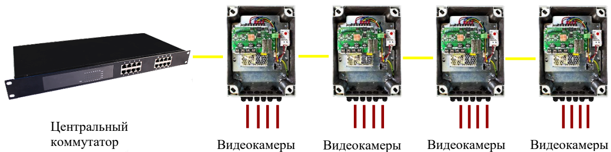
Рисунок 8. Подключение коммутаторов в топологию «линия»
