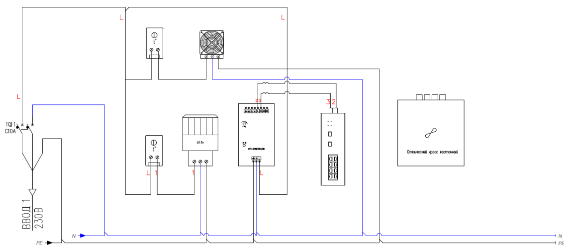
Рисунок 1 – Устройство шкафа
