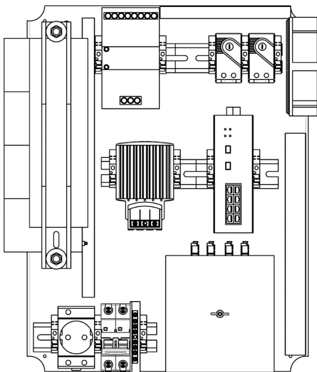
Рисунок 1 – Устройство шкафа
