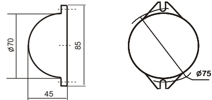
Рис.1. Габаритные и установочные размеры оповещателя
