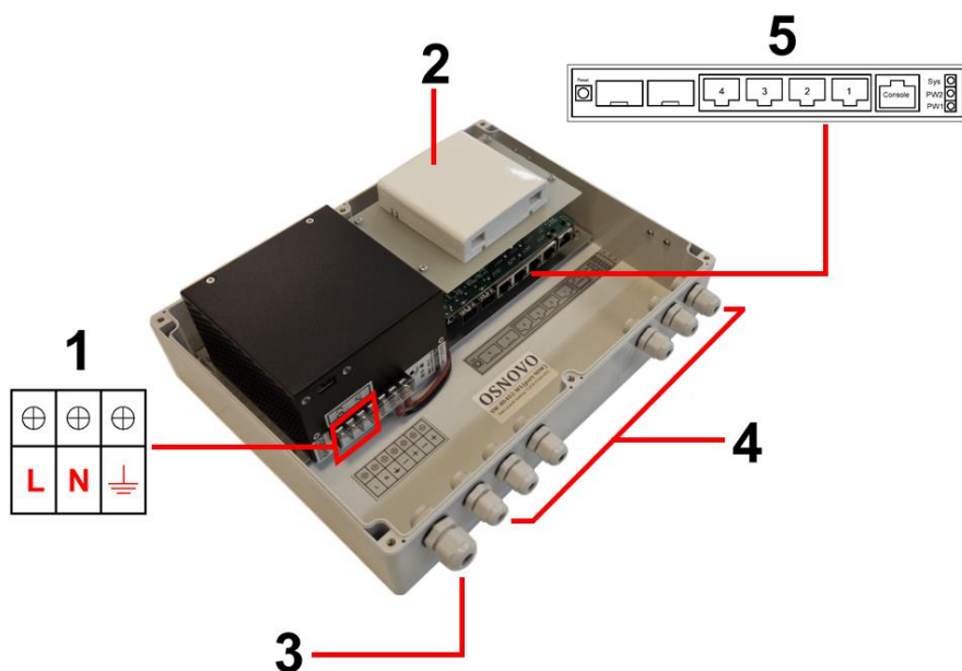
Рис.4 Подключение уличного коммутатора SW-80402-WL(port 90W).
