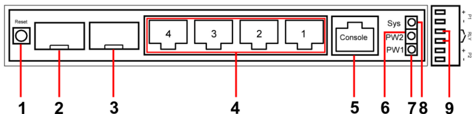
Рис.3 Уличный коммутатор SW-80402-WL(port 90W), разъемы, кнопки и индикаторы.
