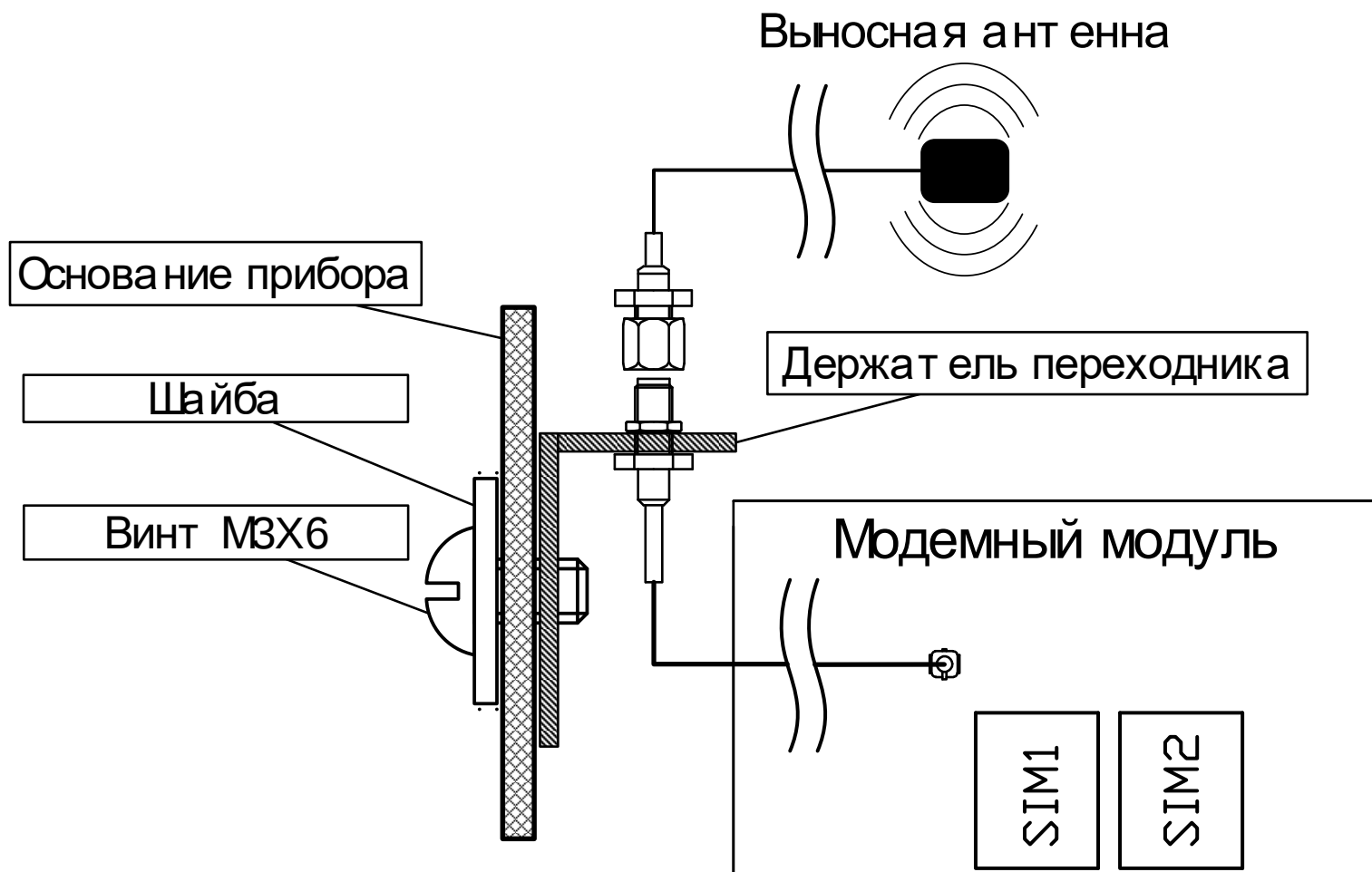
Рисунок 1. Схема монтажа Антенны GSM с переходником
