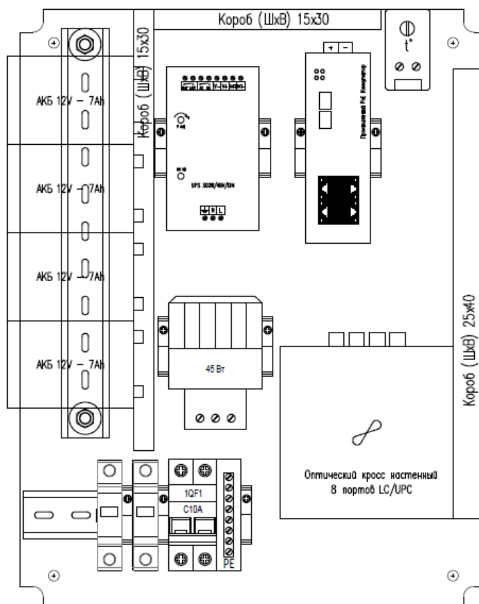
Рисунок 1 – Устройство шкафа
