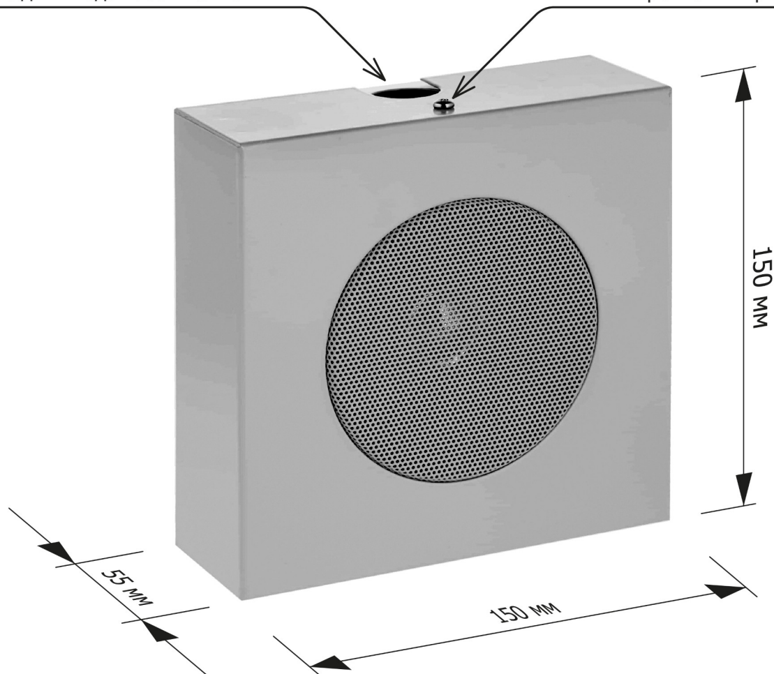
Рис.4 Габаритные размеры БА
