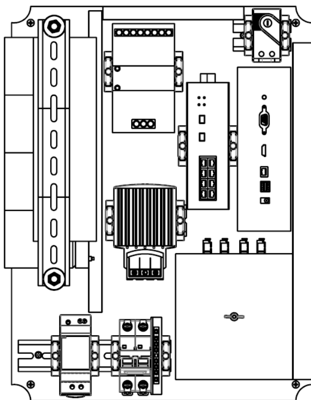
Рис. 10 – Расположение элементов на монтажной плате
