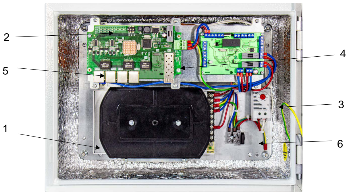
Рис. 6. Расположение составных частей Релион-SW-M-1G-1/4PoE+/60W
