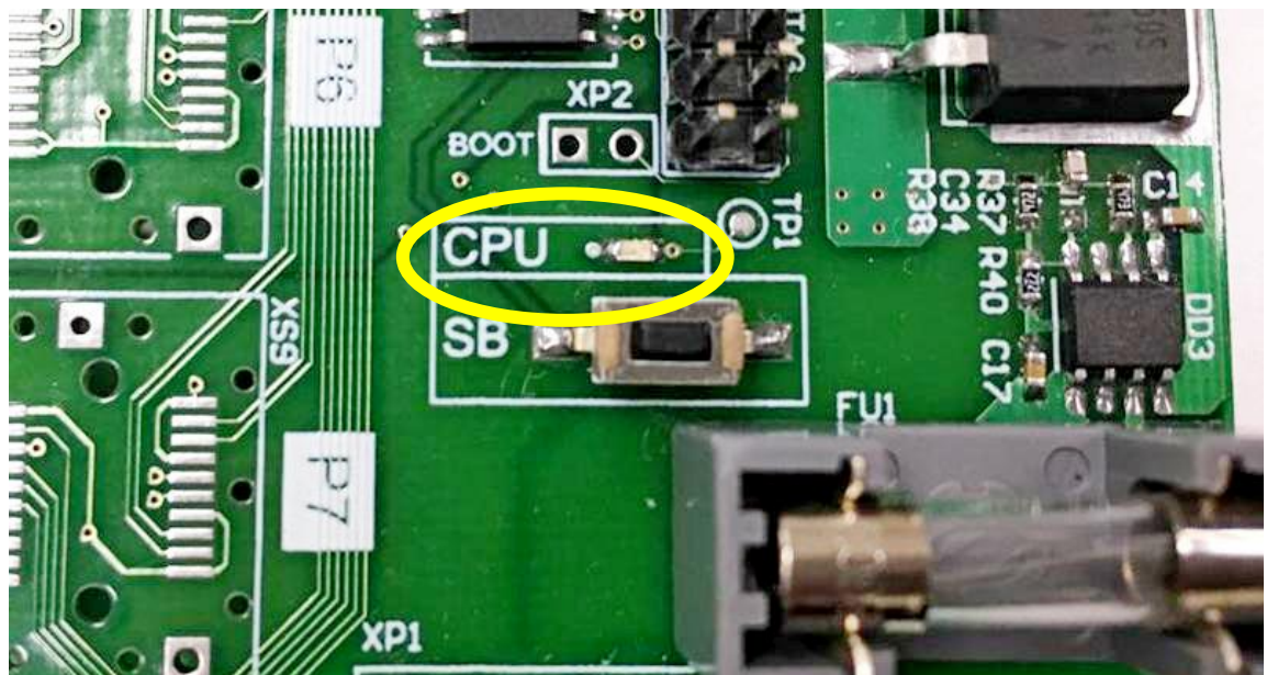
Рисунок 12. Расположение элементов индикации и настройки на плате коммутатора
