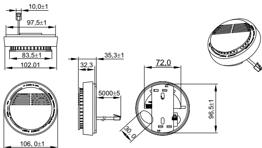
Рисунок 5 – Датчик задымления / Figure 5 – Smoke sensor
