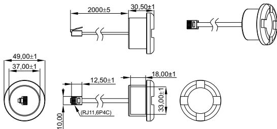
Рисунок 4 – Датчик воды / Figure 4 – Water sensor
