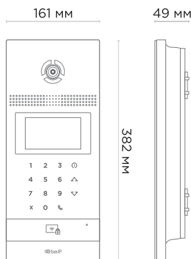
Вызывная панель
