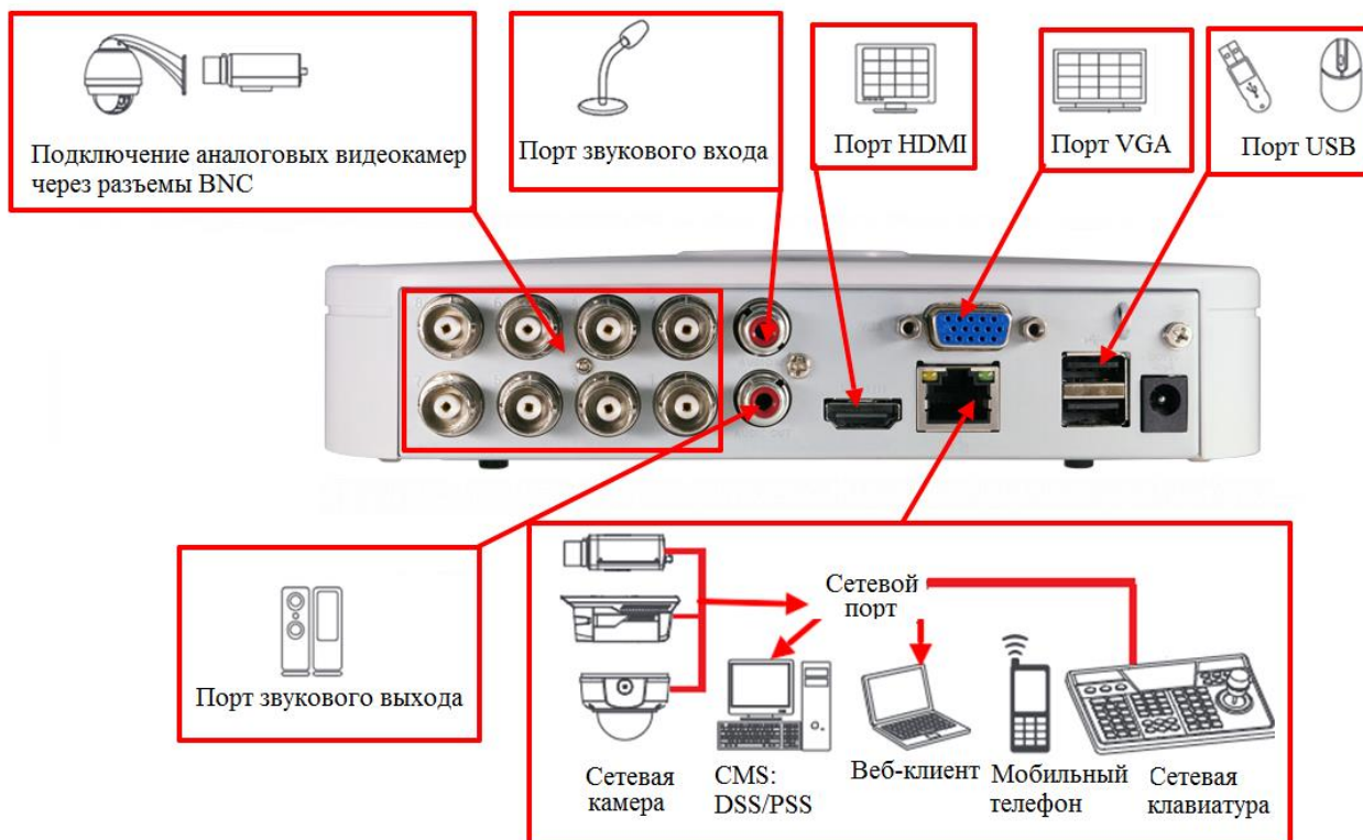
Рисунок 4.2 Внешний вид задней панели
