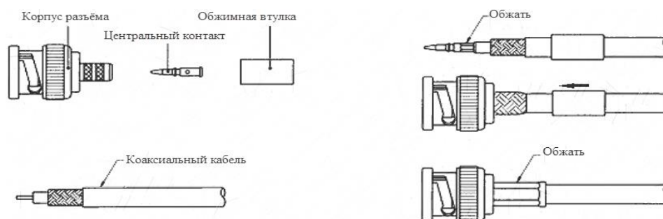
Рисунок 5.1 Схема обжима BNC
