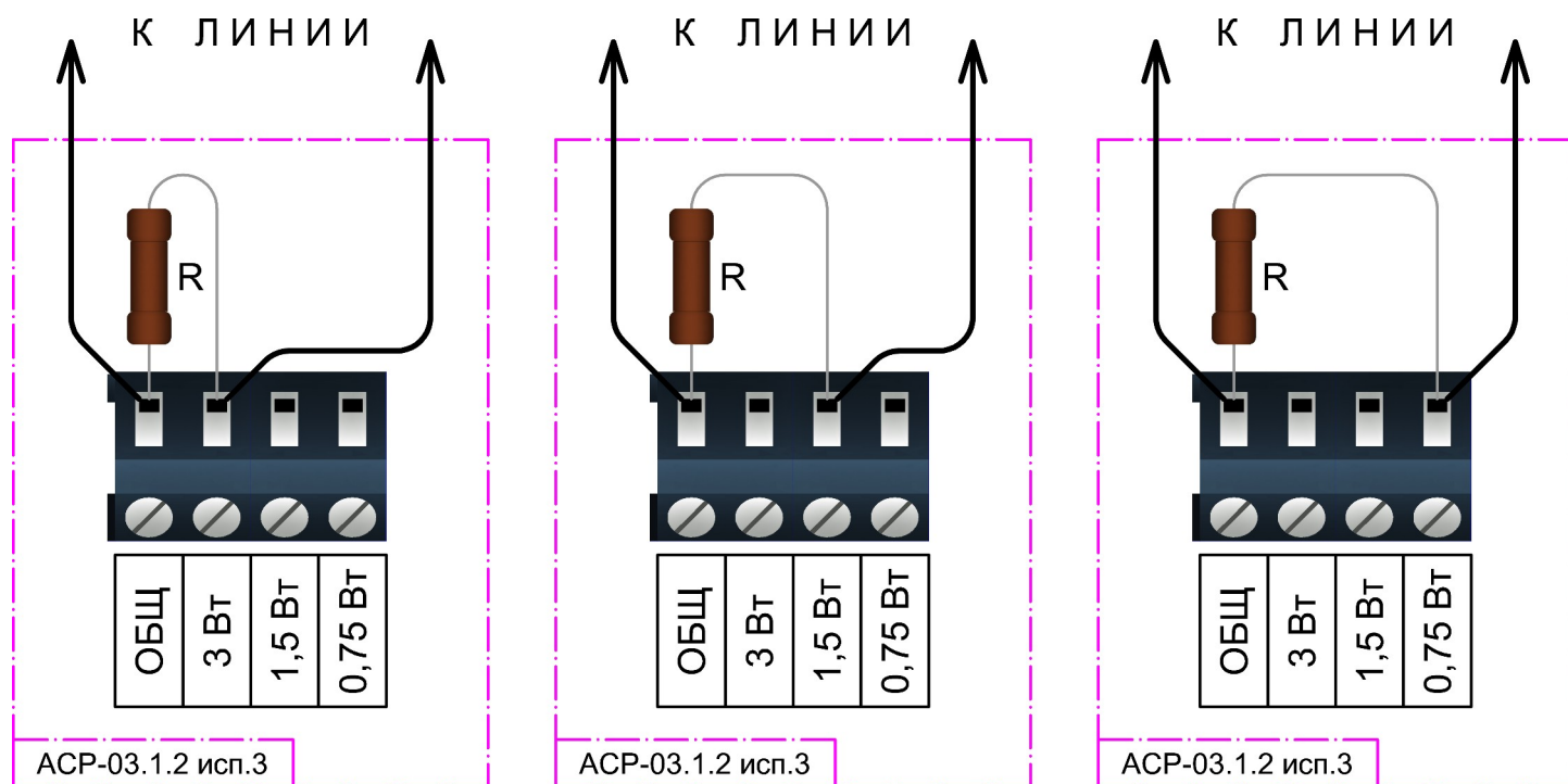
Рис.3 Схема подключения нагрузочного резистора к БА исполнения 3 согласно выбранной мощности
