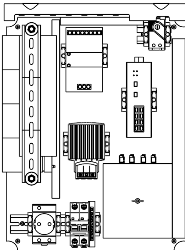
Рисунок 1 – Устройство шкафа
