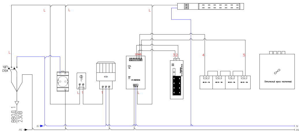
Рисунок 2 – Схема электрическая принципиальная
