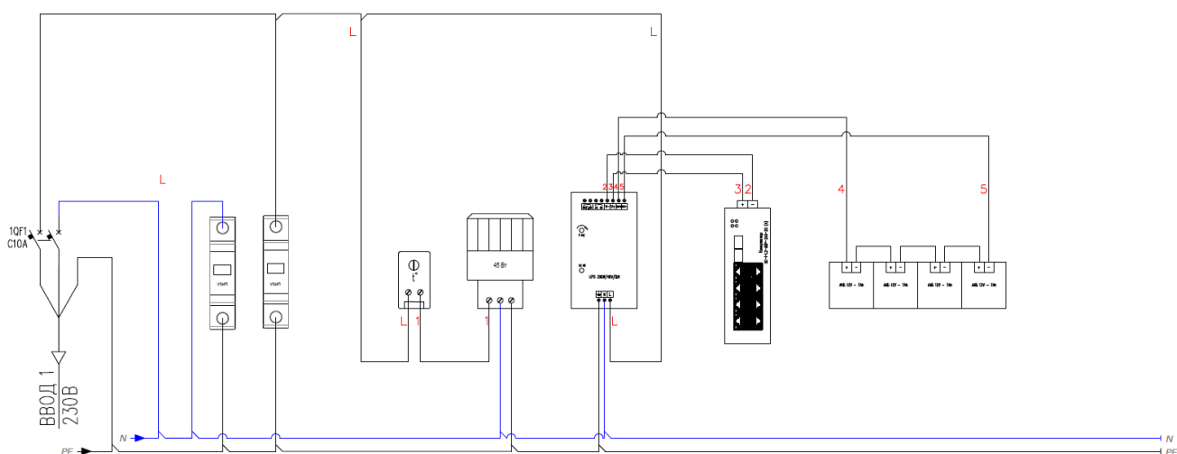
Рисунок 1 – Устройство шкафа
