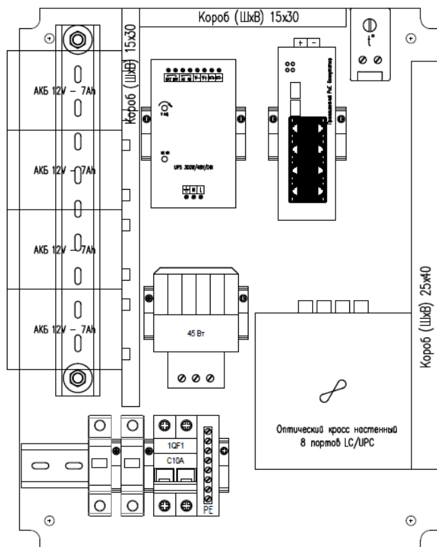
Рисунок 1 – Устройство шкафа
