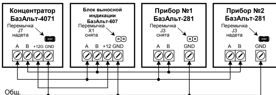
Рисунок 2 – Пример подключения расширителей к прибору
