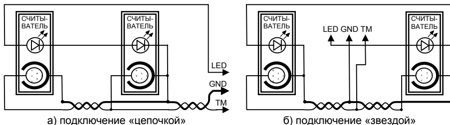
Рисунок 10 – Подключение двух считывателей
