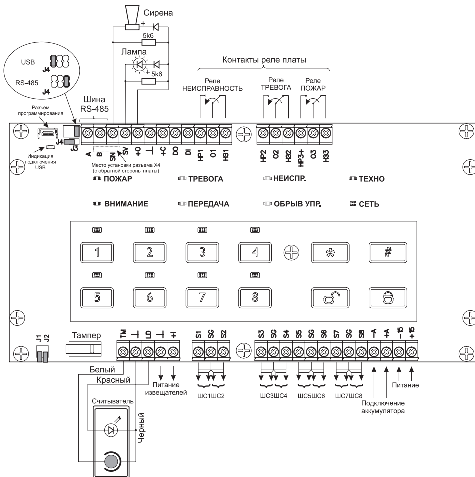
Рисунок 11 – Монтажная схема прибора
