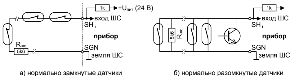
Рисунок 7 – Примеры монтажа охранных шлейфов
