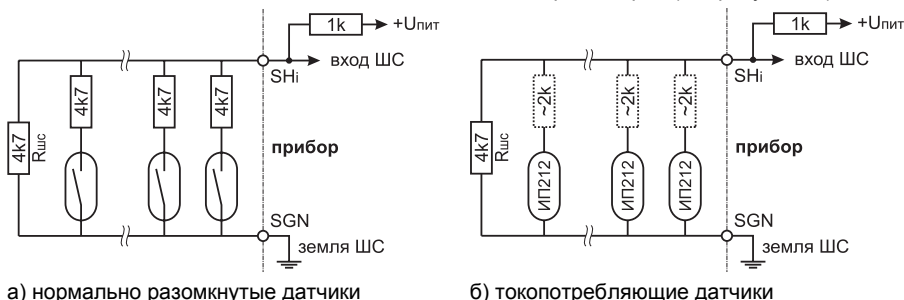
Рисунок 9 – Примеры монтажа пожарных двухпороговых шлейфов
