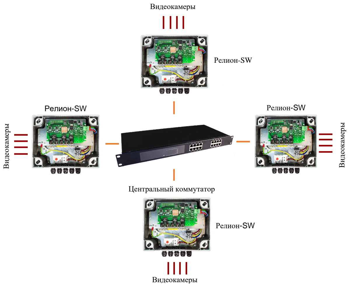
Рисунок 10. Подключение коммутаторов в топологии «звезда»
