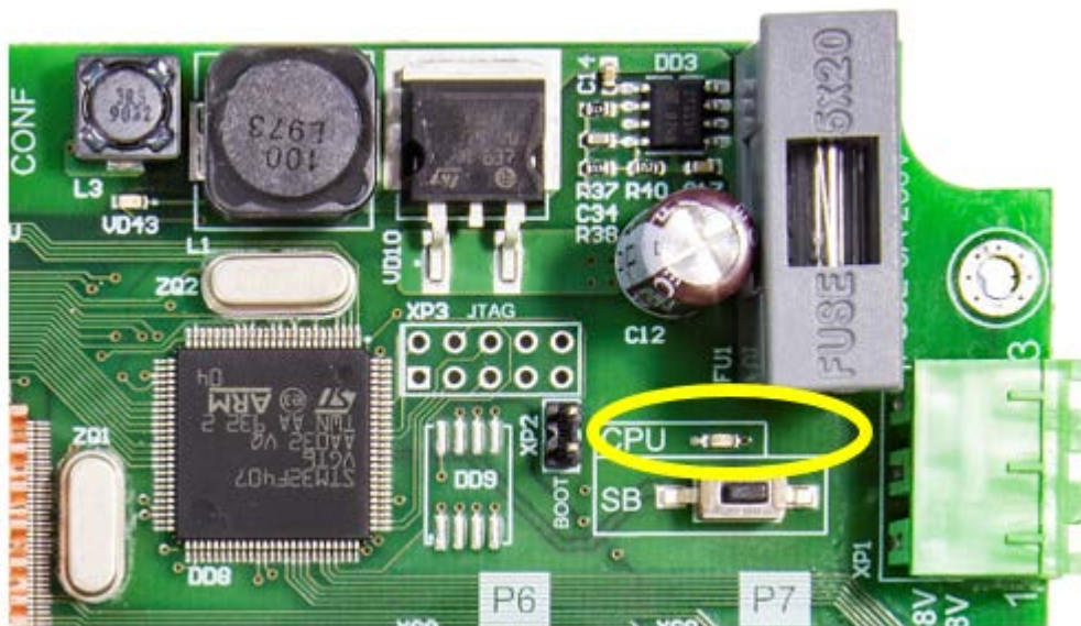
Рисунок 13. Расположение элементов индикации и настройки на плате коммутатора
