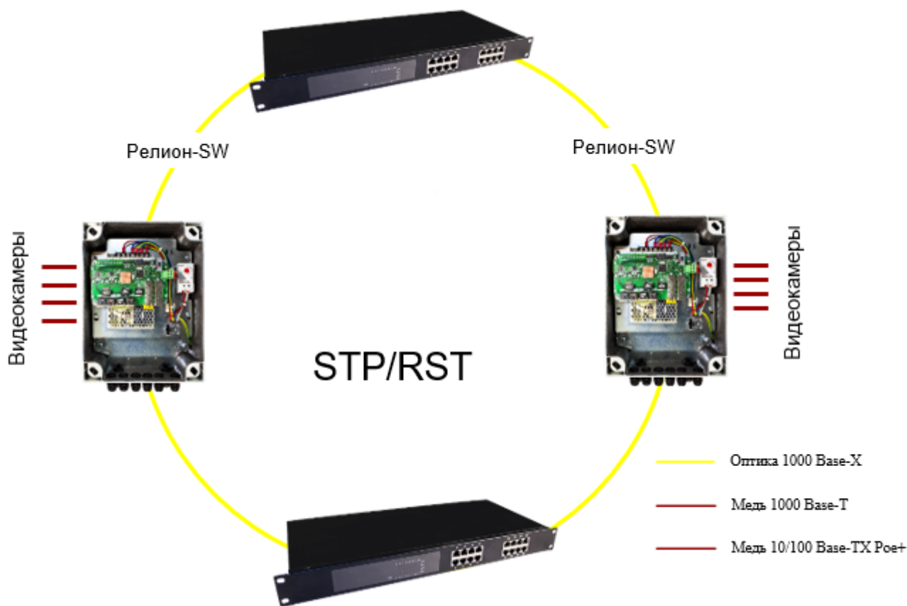
Рисунок 12. Подключение коммутаторов в топологию «кольцо»
