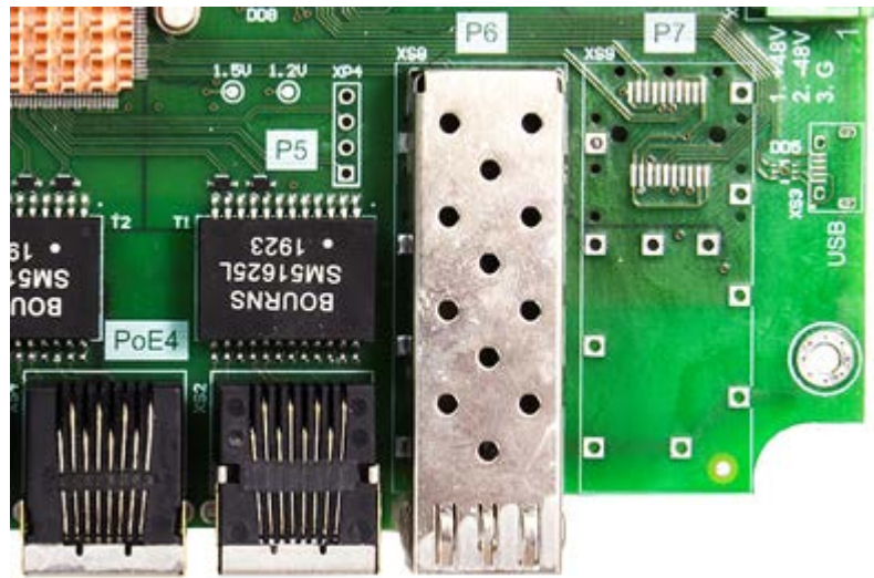
Рисунок 9. Фото порта SFP Коммутатора Топология подключения коммутаторов в сеть:
