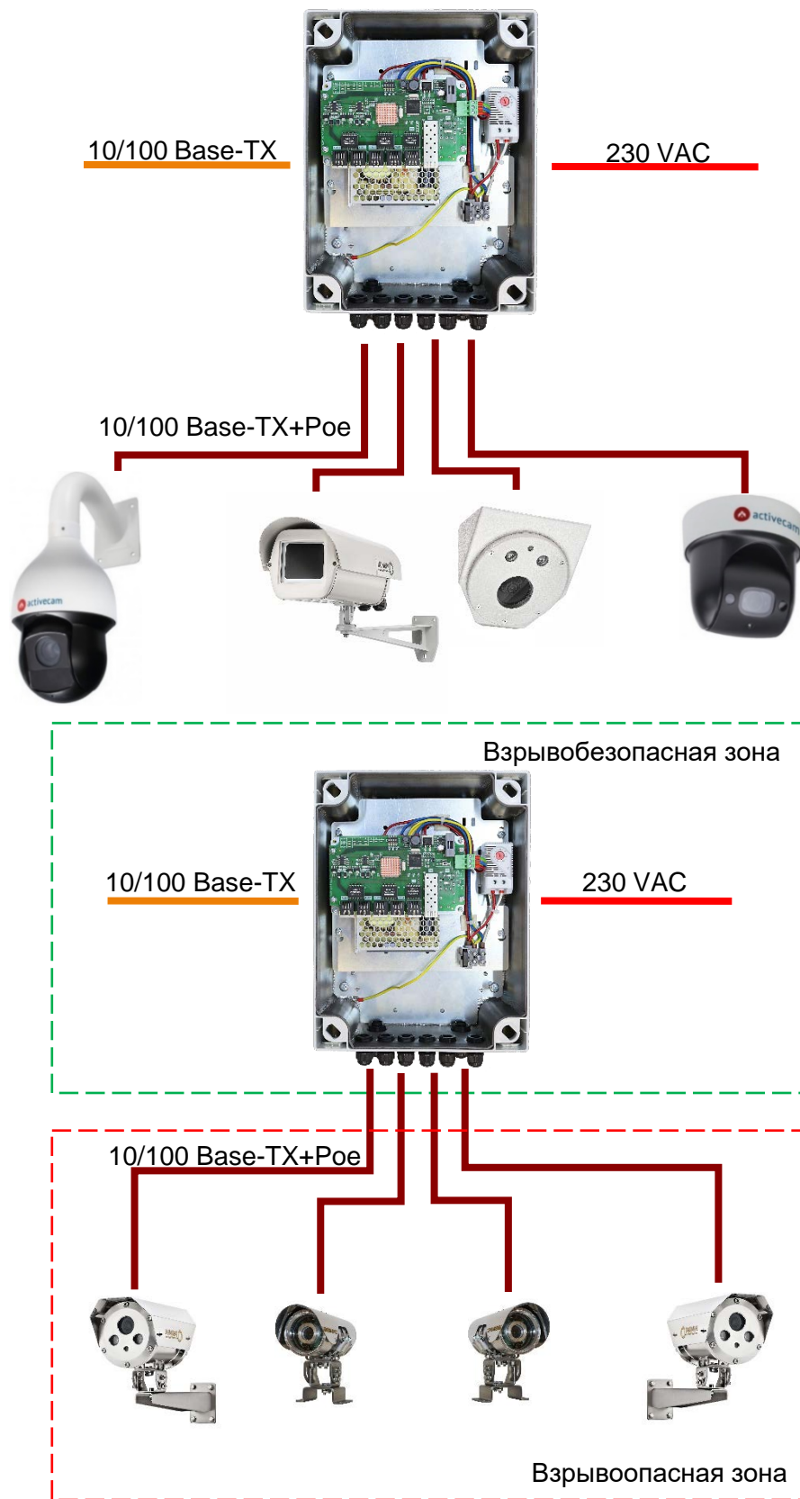
Рисунок 1. Типовые схемы подключения коммутаторов по медному кабелю.
