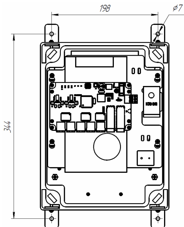
Рисунок 15. Расположение крепежных элементов коммутатора
