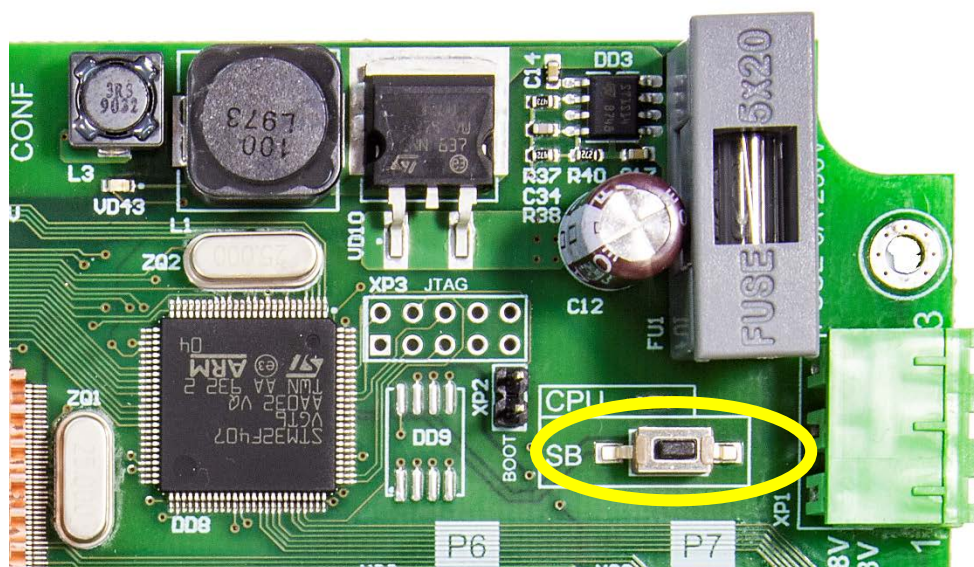
Рисунок 14. Кнопка сброса настроек коммутатора на заводские установки
