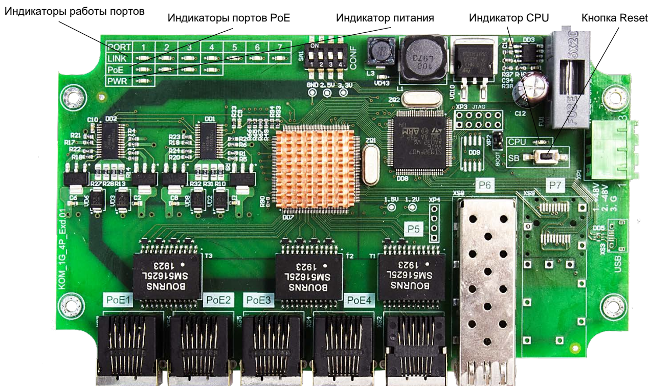
Рис. 7. Расположение элементов на плате коммутатора.
