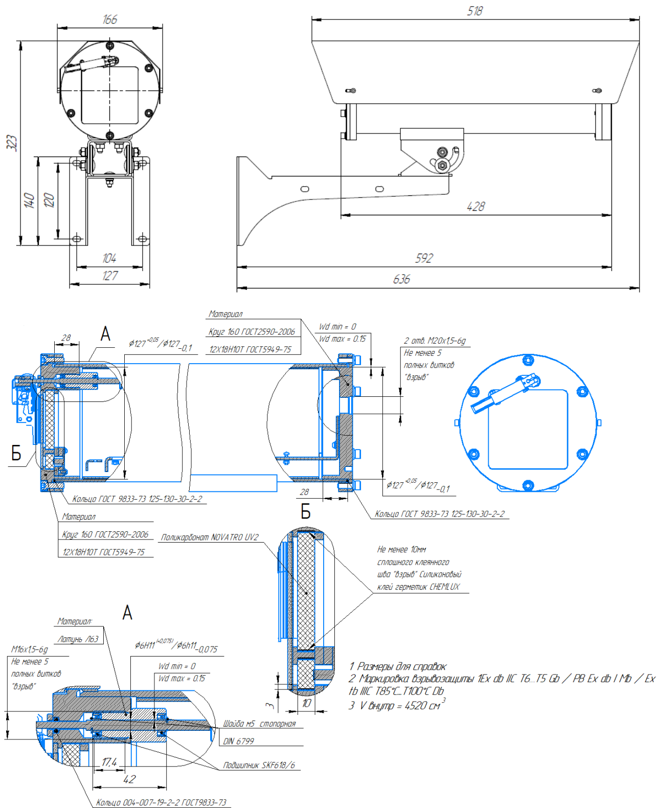
Рисунок А2 – Габаритные размеры термокожуха с крепежно-юстировочным устройством и чертеж безопасности Релион-ТКВ-400-Н-ИК-СО
